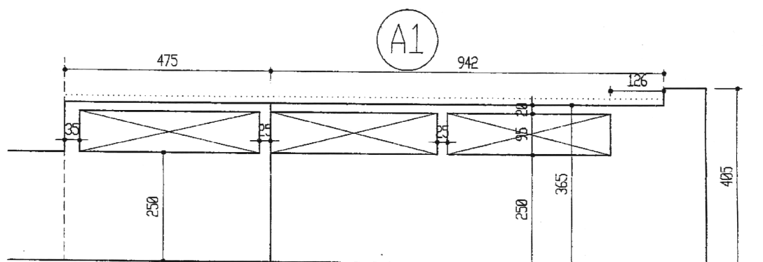
(圍牆)立面圖
